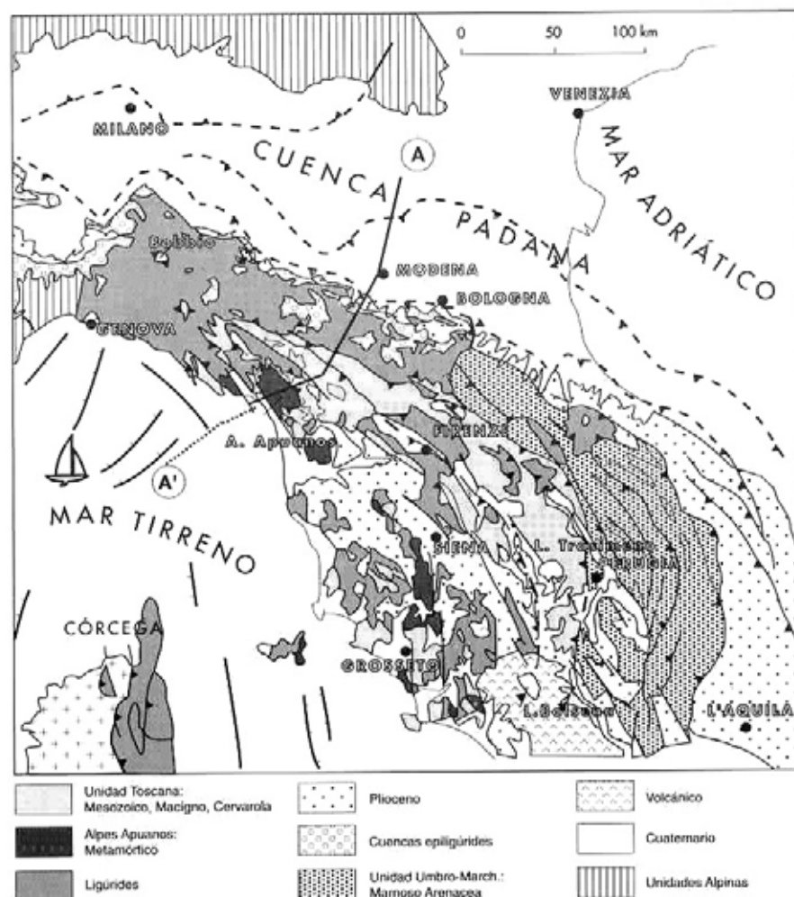
Fig. 2.— Mapa esquemático de la parte septentrional de la península Itálica y situación del corte basado en el mapa tectónico de Italia (CNR, 1991) y otras fuentes.
